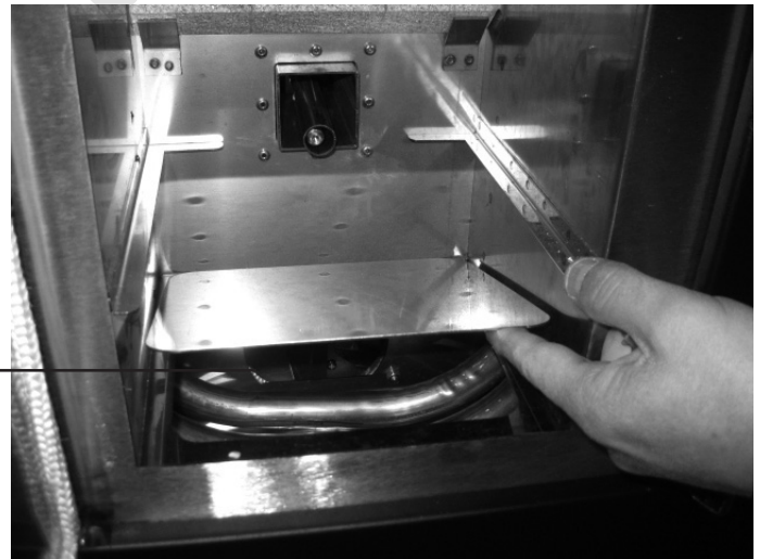
Tubos de intercambio superior
